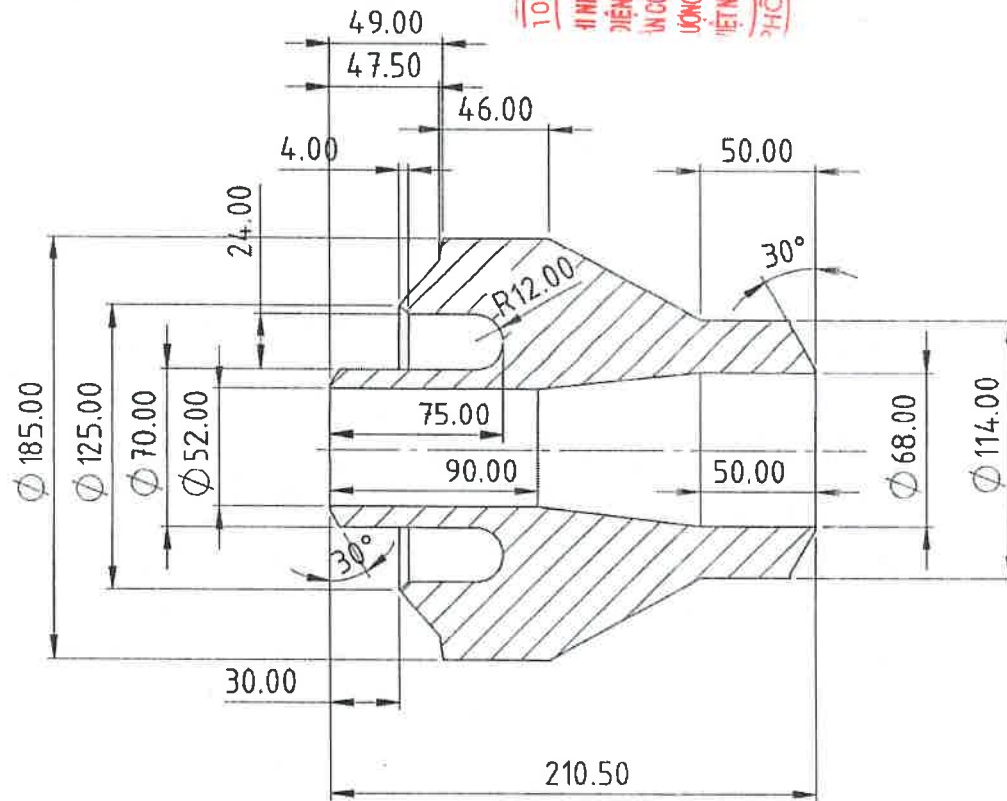
SECTION B-B SCALE 1 : 3
