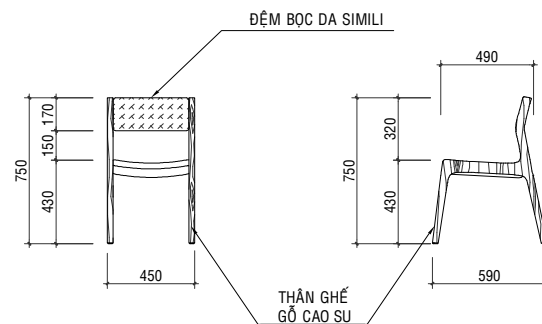
MẶT ĐỨNG
