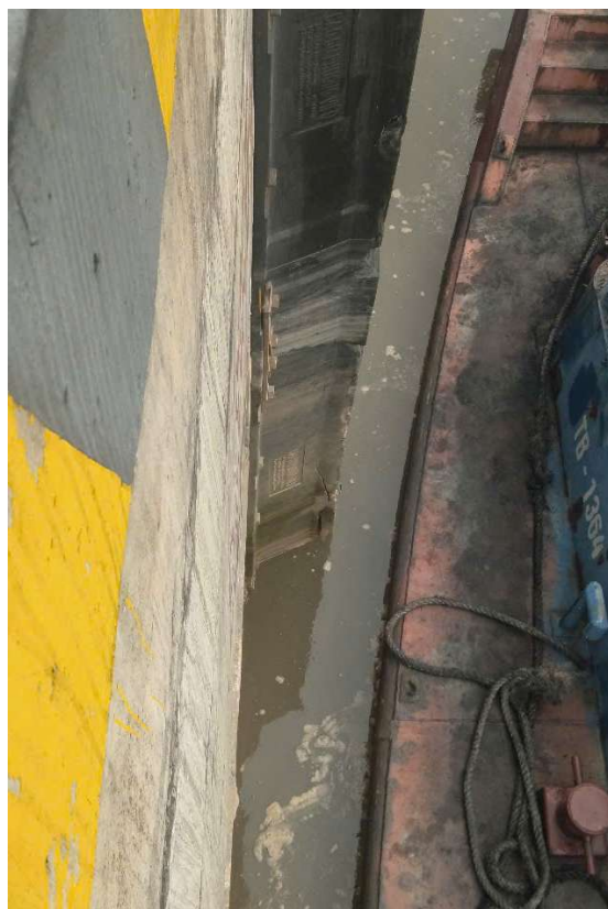
Đệm va số II-5D
